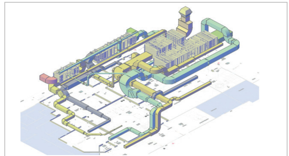
3- dimensionale Darstellung der Lüftungsanlagen
